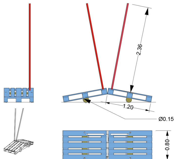
MOUVEMENT DES PALETTES À PARTIR D'UN RONDIN DE 15 CM DE DIAMÈTRE
